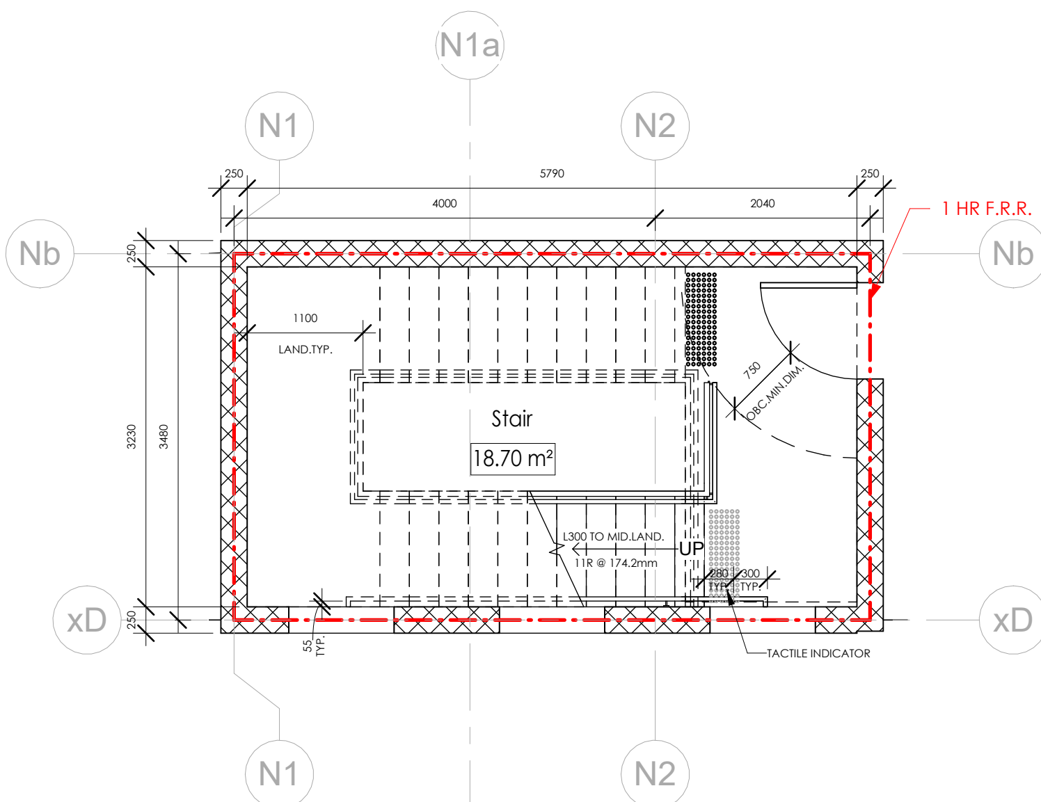
2 L300 Stair Plan 1 : 50
