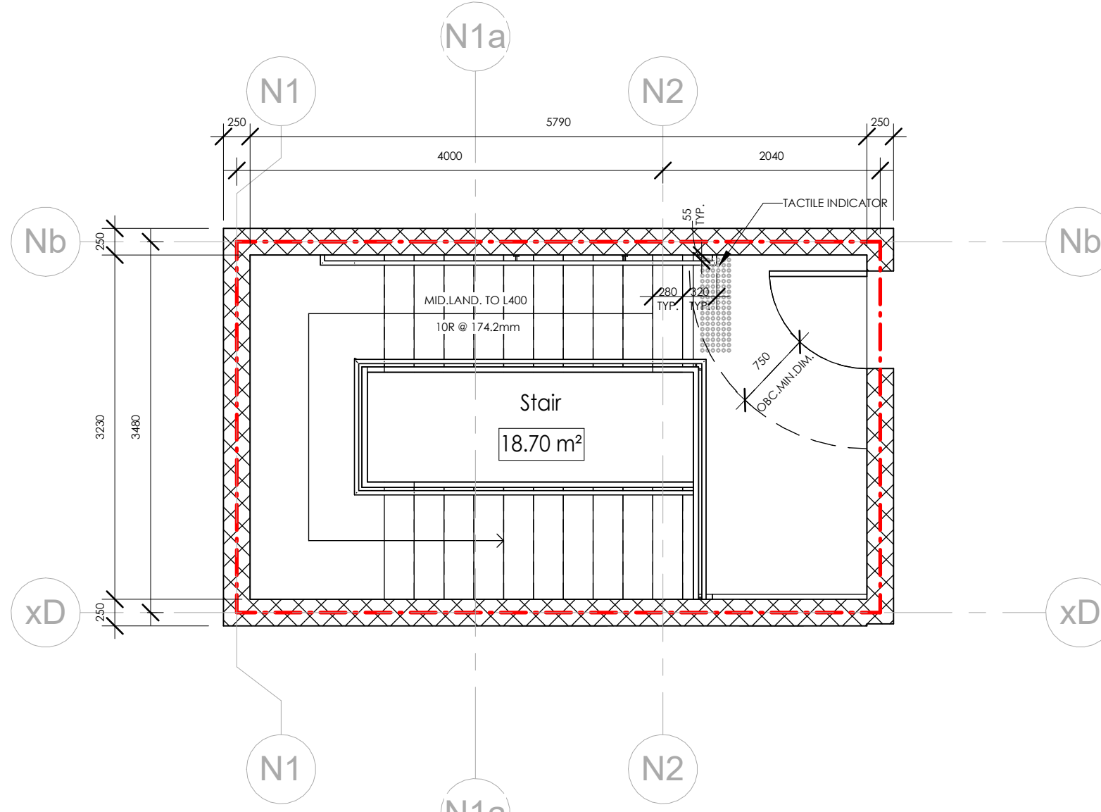
3 L400 Stair Plan 1 : 50
