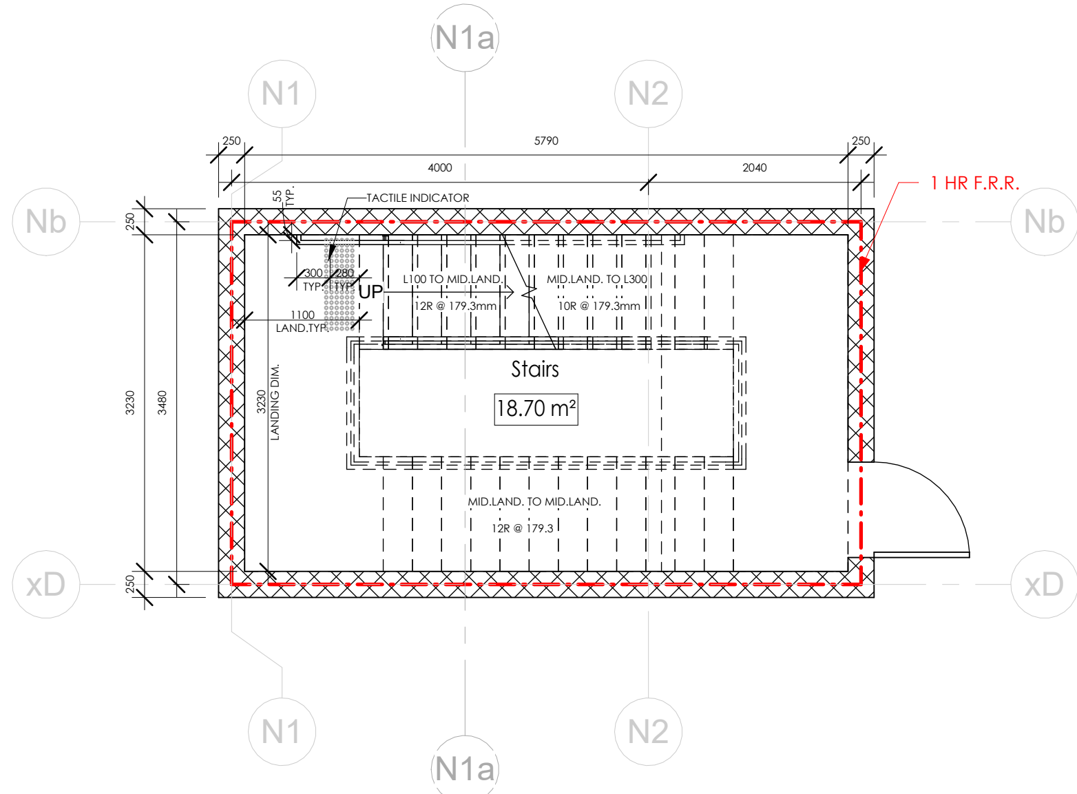
1 L100 Stair Plan 1 : 50
