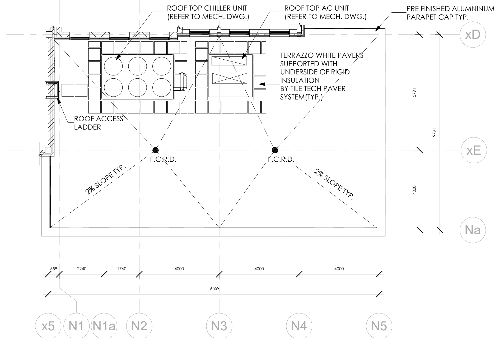
6 L300 ROOF PLAN 1 : 100
